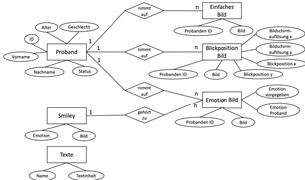
Abbildung 3.1: ER-Modell über den grundlegenden Aufbau der Datenbank und der Tabellen
