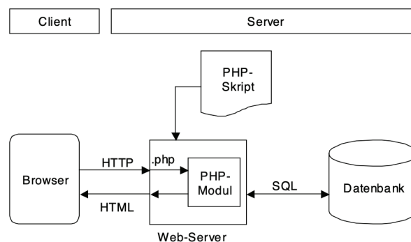
Abbildung 2.5: Ablauf und Funktionsweise einer Datenbankabfrage über PHP [BvM01]
